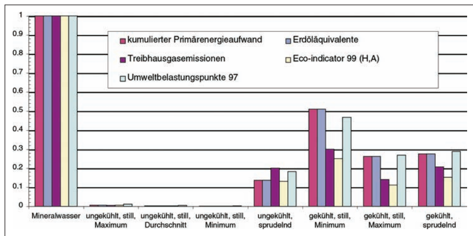
Abb. 2 Relativer Vergleich der Umweltbelastungen von Mineralwasser und Hahnenwasser. Die Höhe des Balkens gibt die Umweltbelastungen der Hahnenwasservariante im Vergleich zur entsprechenden Variante für Mineralwasser an.
